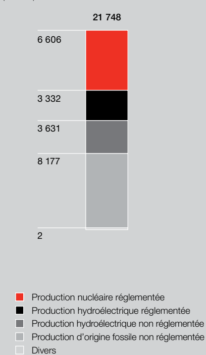
Capacité de production en service par secteur 31 décembre 2008 (en MW)
