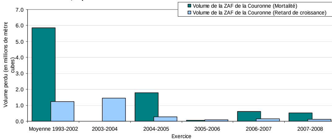
Figure 3d – Estimation de pertes en volume des terres de la Couronne dans la ZAF, imputables aux insectes forestiers
