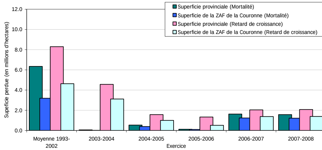
Figure 3c – Estimation de la superficie perturbée par les insectes forestiers
