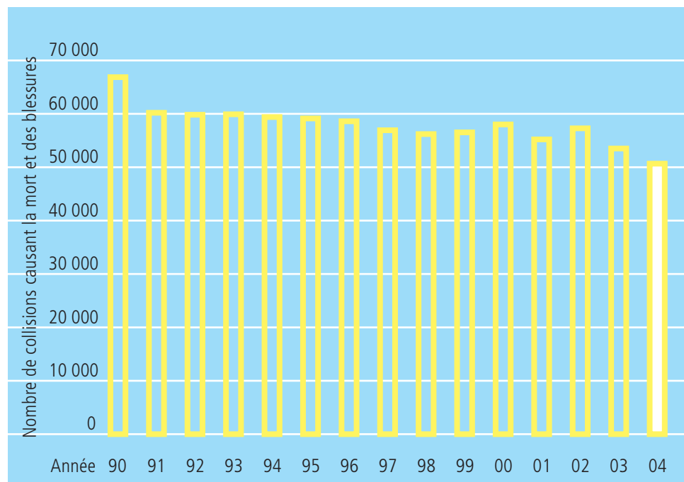
Figure 1 | Nombre total de collisions ayant causé la mort et des blessures en Ontario, 1990 à 2004
