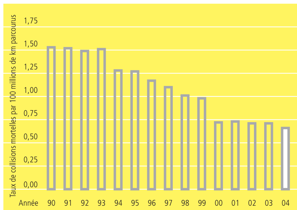
Figure 3 | Taux de collisions mortelles par 100 millions de kilomètres parcourus en Ontario, 1990 à 2004
