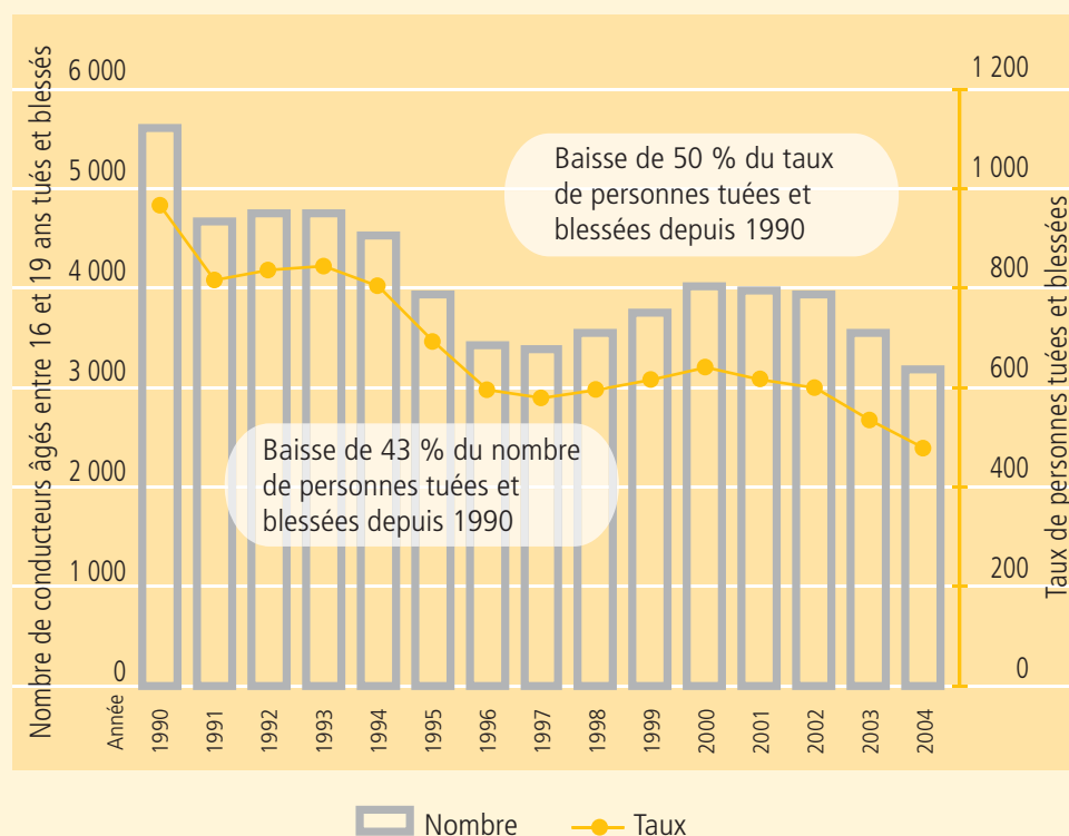
Nombre et taux* de conducteurs âgés entre 16 et 19 ans tués et blessés : 1990–2004
