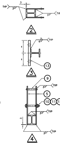
4 LUGS DETAIL
