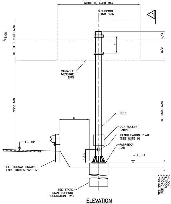
ELEVATION
