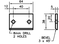
4 LUGS DETAIL
