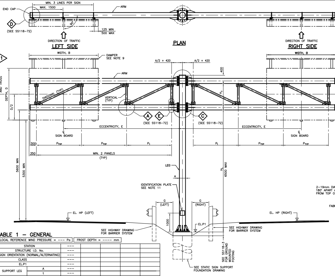
ELEVATION
