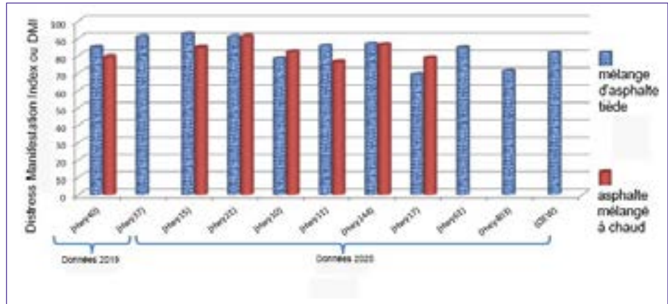
Figure 2 : Données recueillies par l'ARAN et analysées par iVision pour comparer le rendement des sections de contrôle en enrobés à chaud et en enrobés tièdes 9 et 10 ans après la pose. Les enrobés tièdes continuent d'offrir un rendement égal à celui des enrobés à chaud dans le cadre de nombreux contrats. Chaque contact WMA contenait une petite section de test HMA et le reste était WMA.
