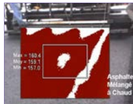
Figure 1a : Image thermique d'asphalte mélangé à chaud montrant des plages de températures allant d'une température minimale de 157,0 °C à une température maximale de 160,4 °C, avec une moyenne de 159,1 °C.
