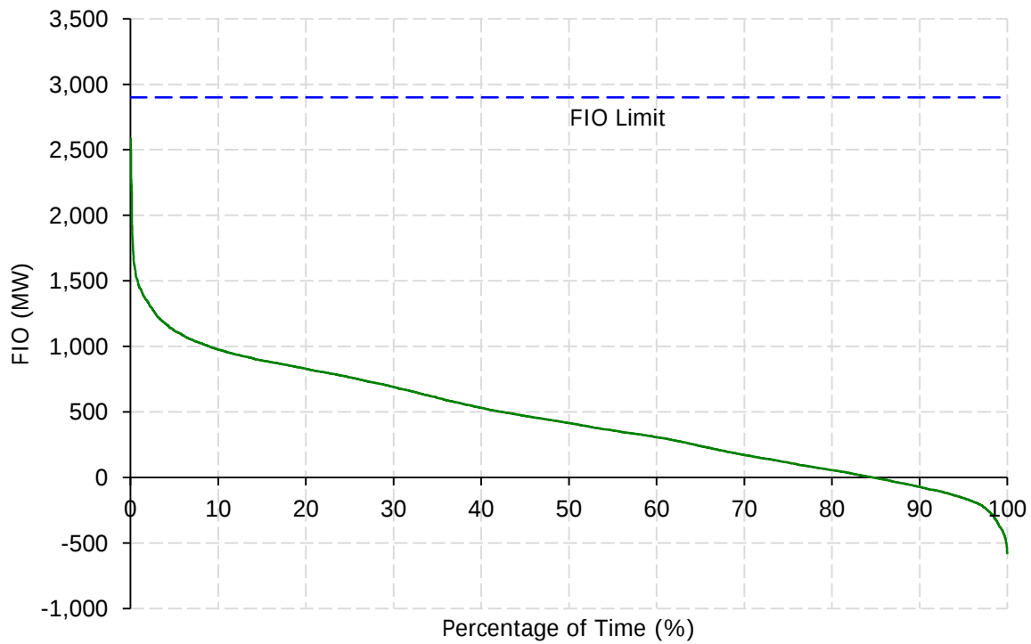
FIO Apr. 1, 2016 to Apr. 1, 2017
