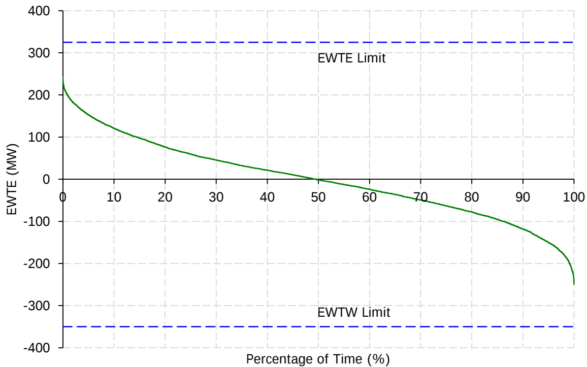
EWTW and EWTE Apr. 1, 2016 to Apr. 1, 2017
