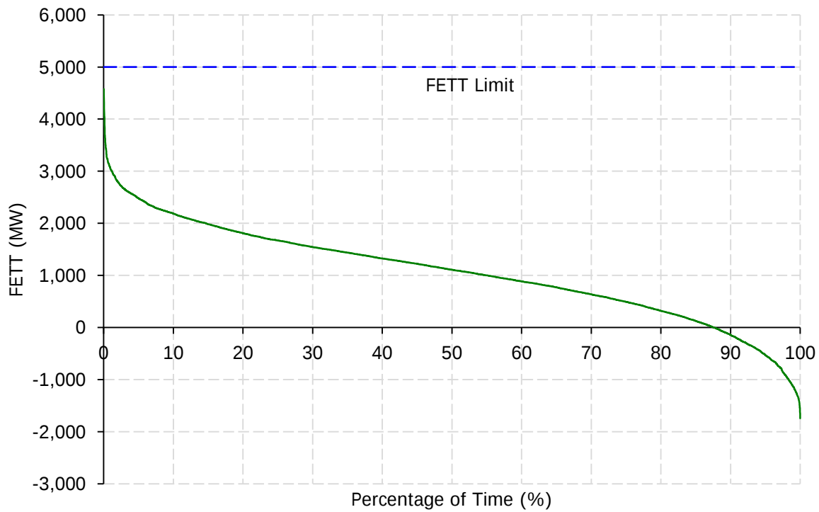
FETT Apr. 1, 2016 to Apr. 1, 2017
