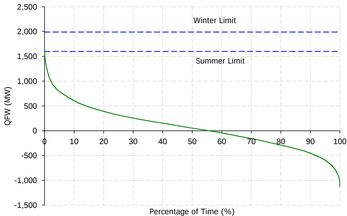
QFW Apr. 1, 2016 to Apr. 1, 2017
