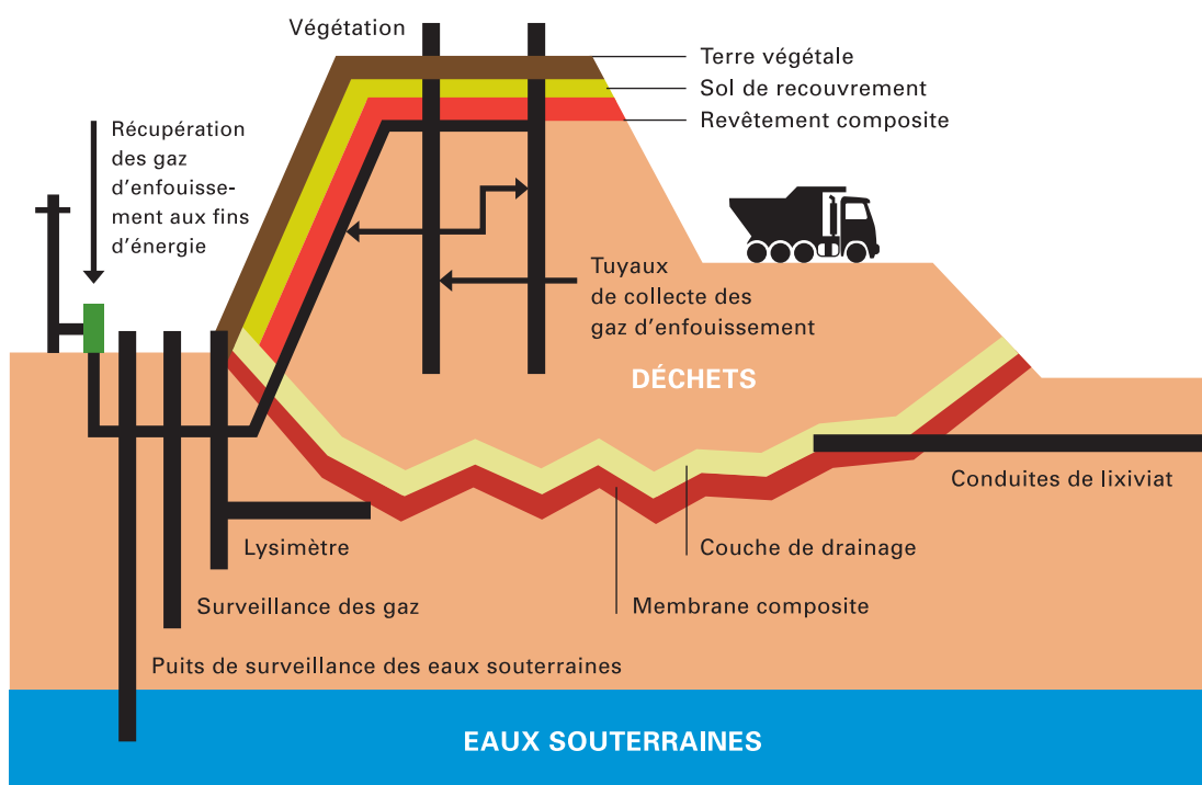
Figure 1 Profil type d'un site d'enfouissement
